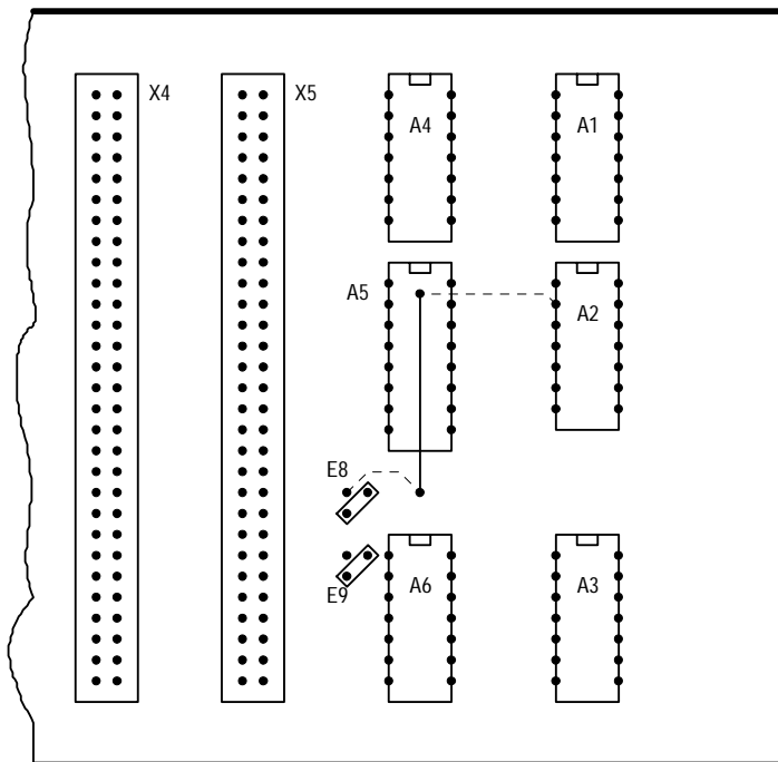
Abb. 4.3 Belegungsplan Busverstärker (Auszug)
