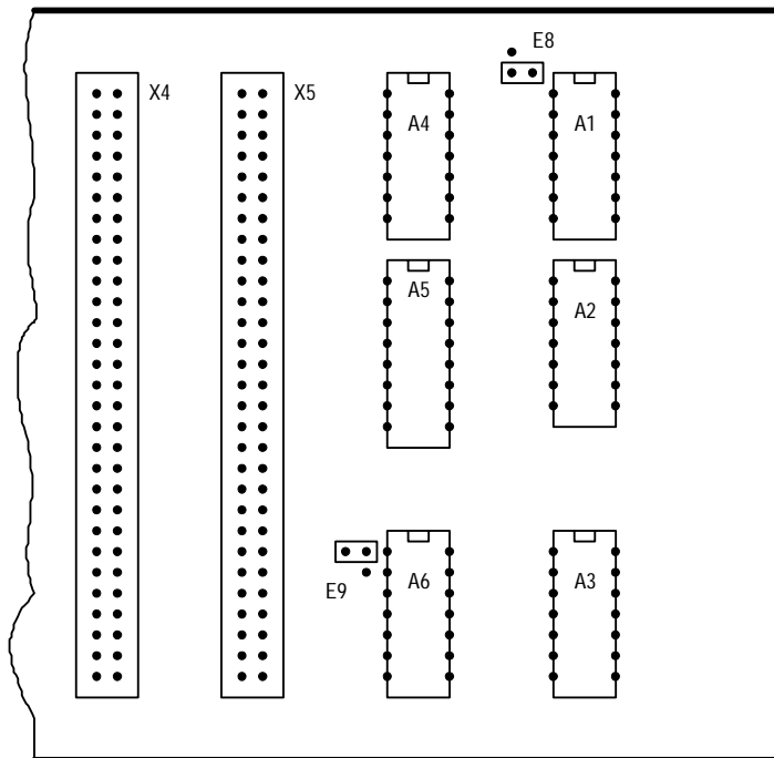
Abb. 4.4 Belegungsplan Busverstärker (Ausschnitt)
