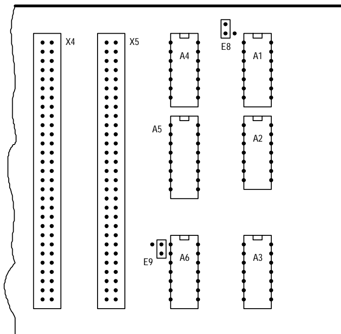
Abb. 4.5 Belegungsplan Busverstärker (Auszug)
