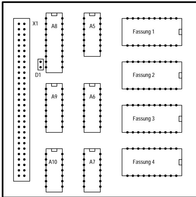
Abb. 4.1 Belegungsplan ROM-Modul
