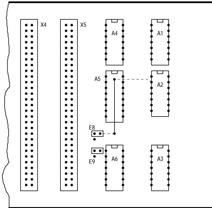
Abb. 4.2 Belegungsplan Busverstärker (Ausschnitt)
